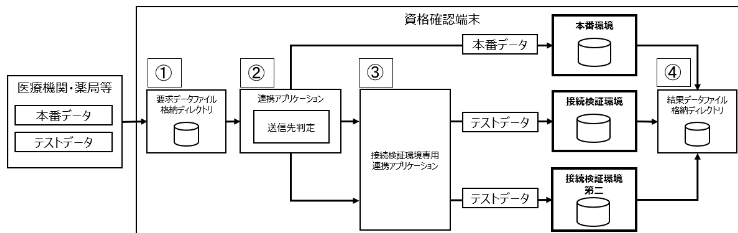
図 7-1 接続検証環境専用連携アプリケーションの処理フロー
